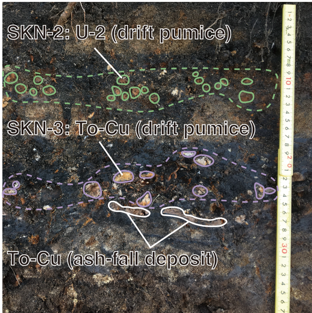
電子付録 S2 U-2 と To-Cu の漂着軽石と To-Cu 降下火山灰のクローズアップ写真 Appendix S2 Closeup photograph of drift pumice of the U-2 and To-Cu tephra, and ash-fall deposit of the To-Cu tephra
