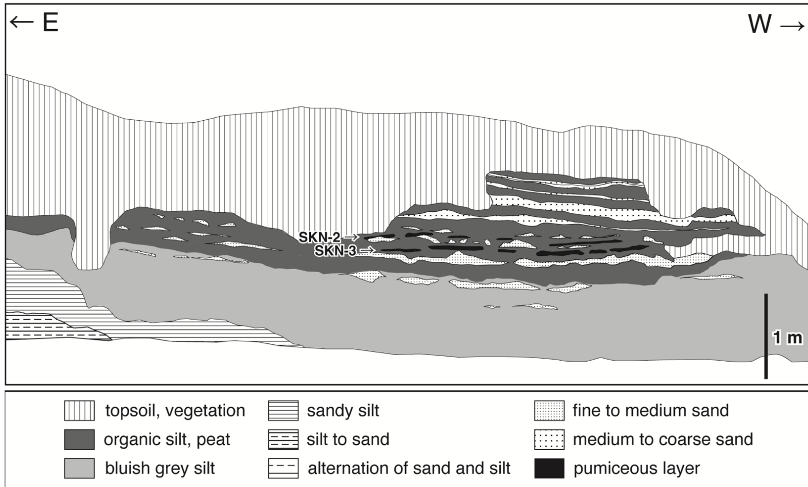
電子付録 S1 露頭のスケッチ Appendix S1 Sketch of the outcrop
